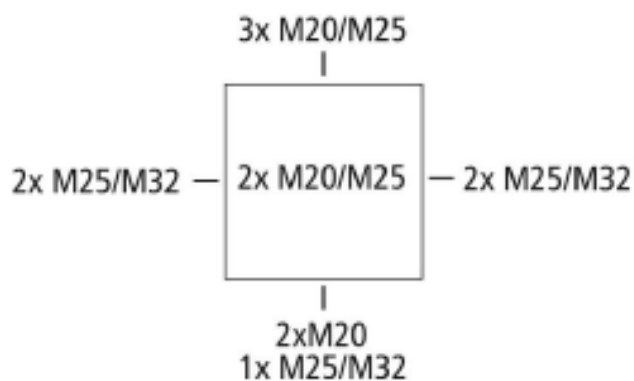
Расположение выбивных отверстий
